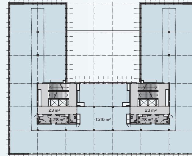
silo plus Regelgeschöß 1-5 Ohne Raumtrennung stehen in einem Regelgeschöß 1.516 m 2 zur Verfügung.
