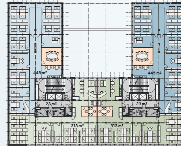
silo plus Regelgeschöß 1-5 Die Regelgeschöße können jeweils auf bis zu vier Einheiten mit zweimal 313 m 2 und zweimal 445 m 2 aufgeteilt werden.
